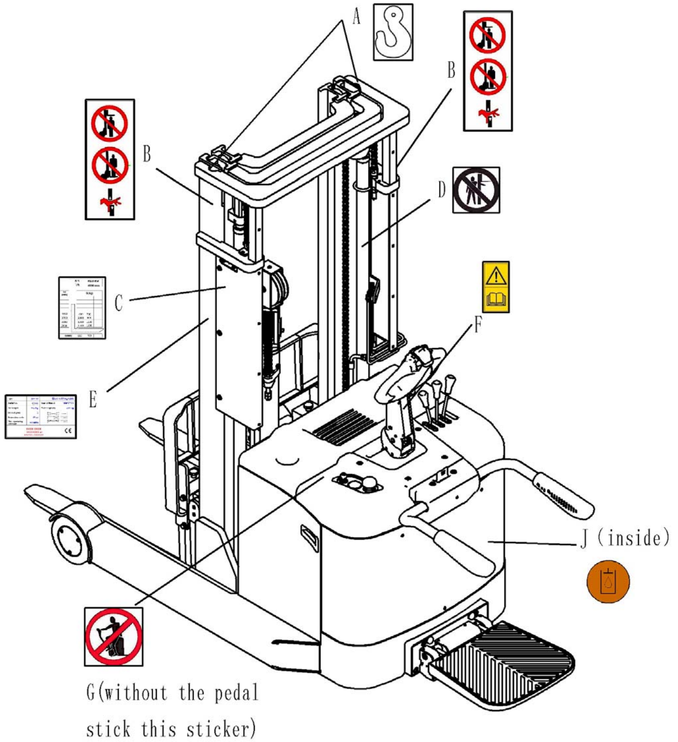
Fig. 2 Sticker (EU)
